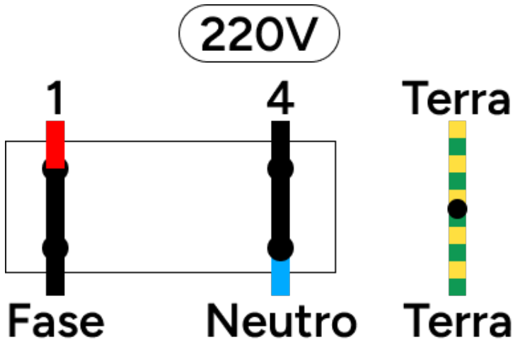
Diagrama 2: Conexões AC (Opcional com trifásico)
