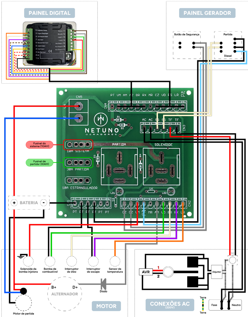
Diagrama 1: Placa elétrica
